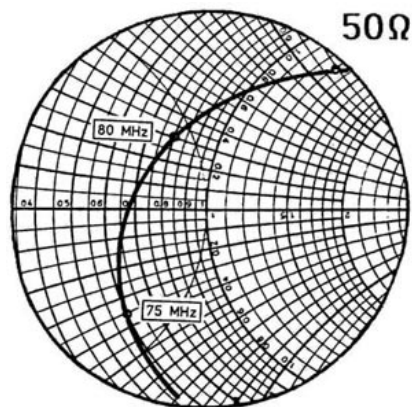
Impedanční charakteristika – 80MHz
